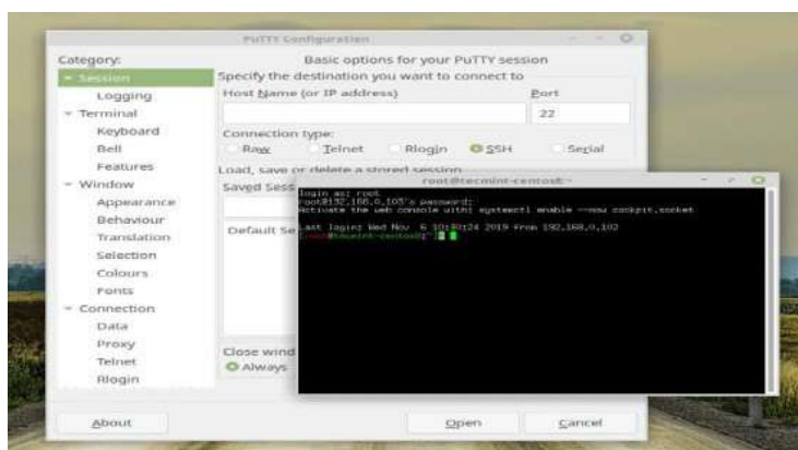
Fig 4 : puTTY sessio
